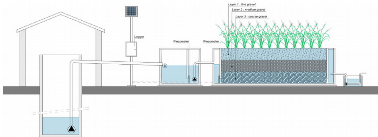
Figura 1. Schema dell'impianto pilota di fitodepurazione sviluppato con il Progetto LIFE PHOENIX.
